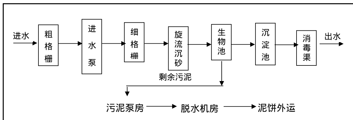
图 5-2-2 CASS 工艺流程图
